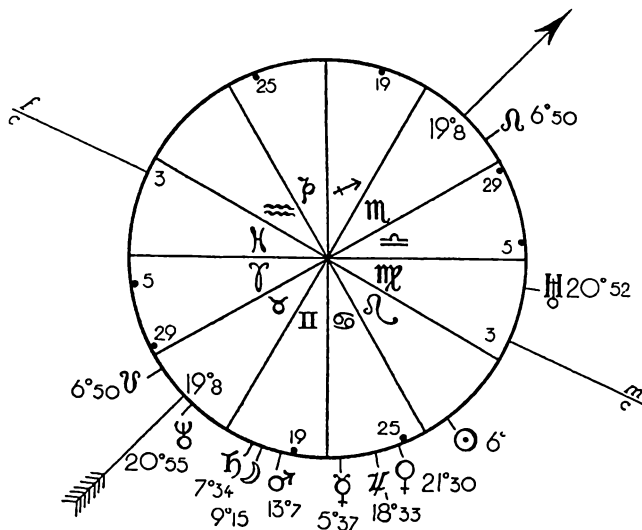
CIEL DE NAISSANCE DE MUSSOLINI
