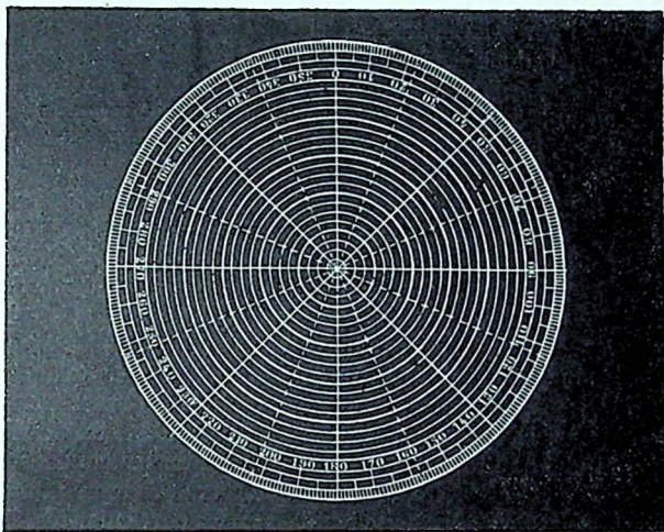
Division du cercle en 360 degrés.
