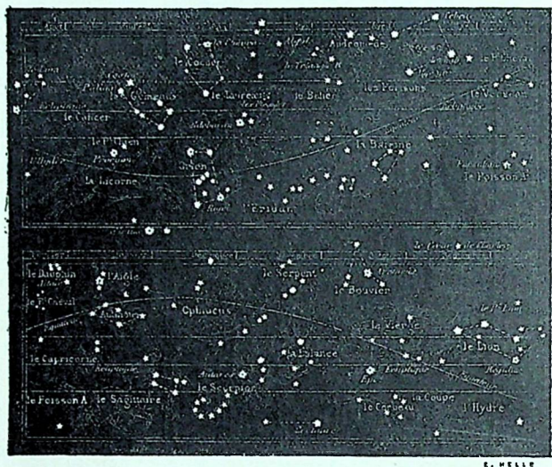
Les Constellations Zodiacales
