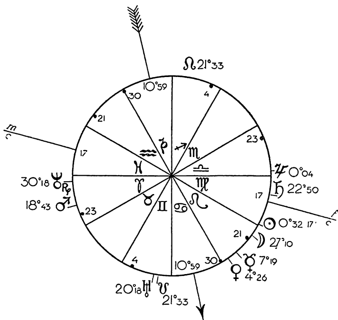
CIEL DE NAISSANCE DE L. BARTHOU
