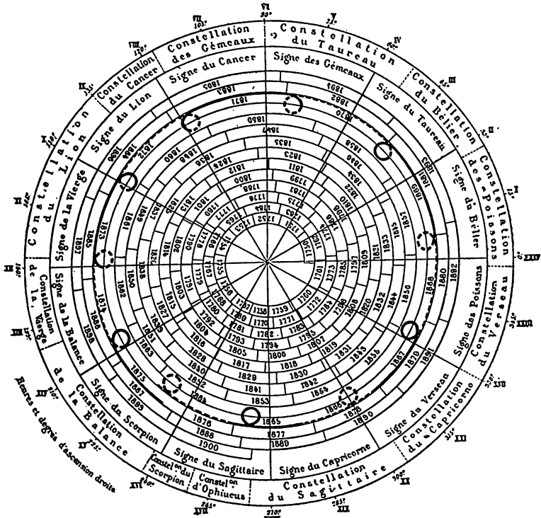
Extrait de l'Astronomie Populaire de Camille Flammarion Mouvement de Jupiter par rapport à la Terre.
