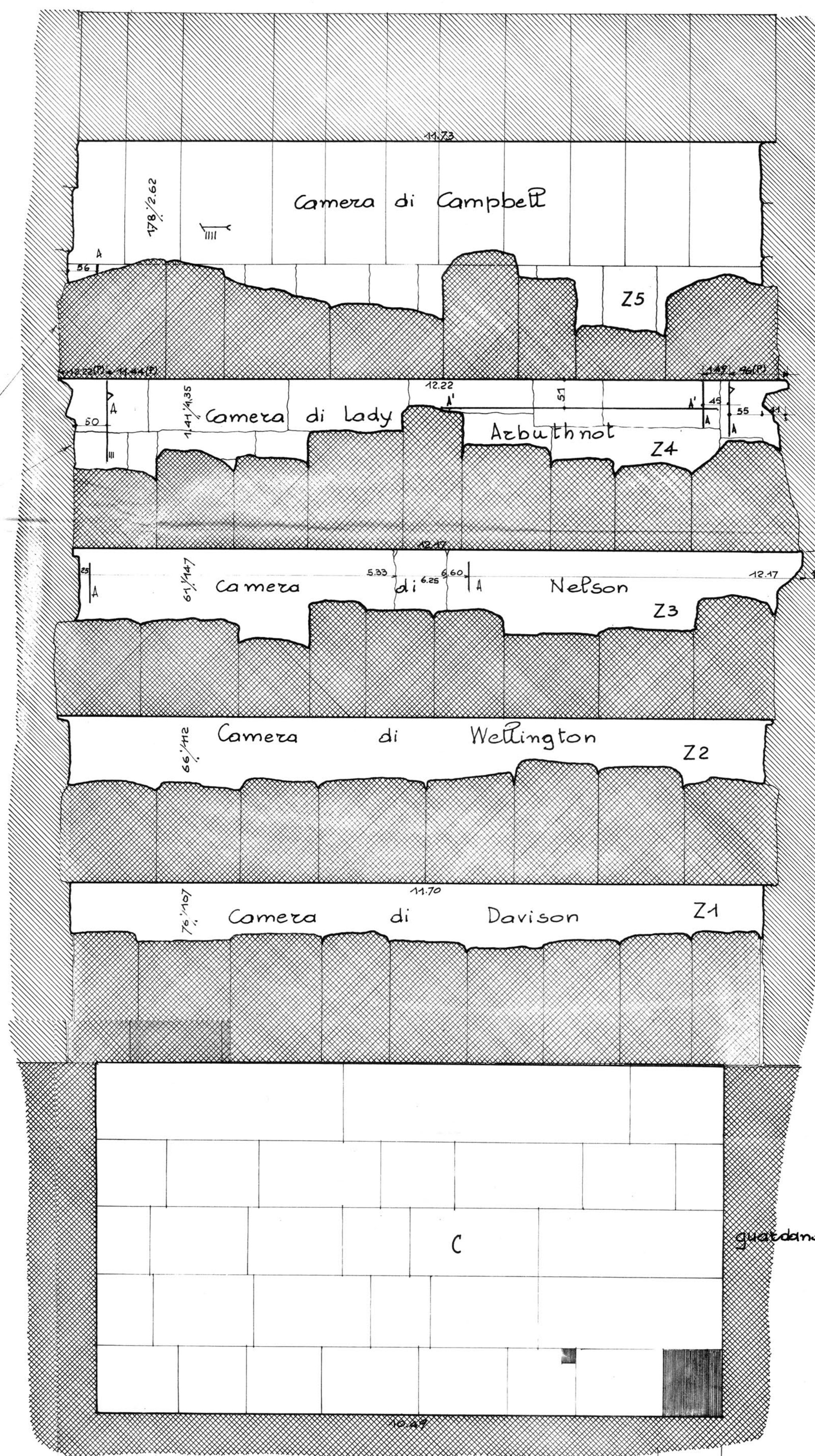
FIG. 3 SEZIONE W-E
