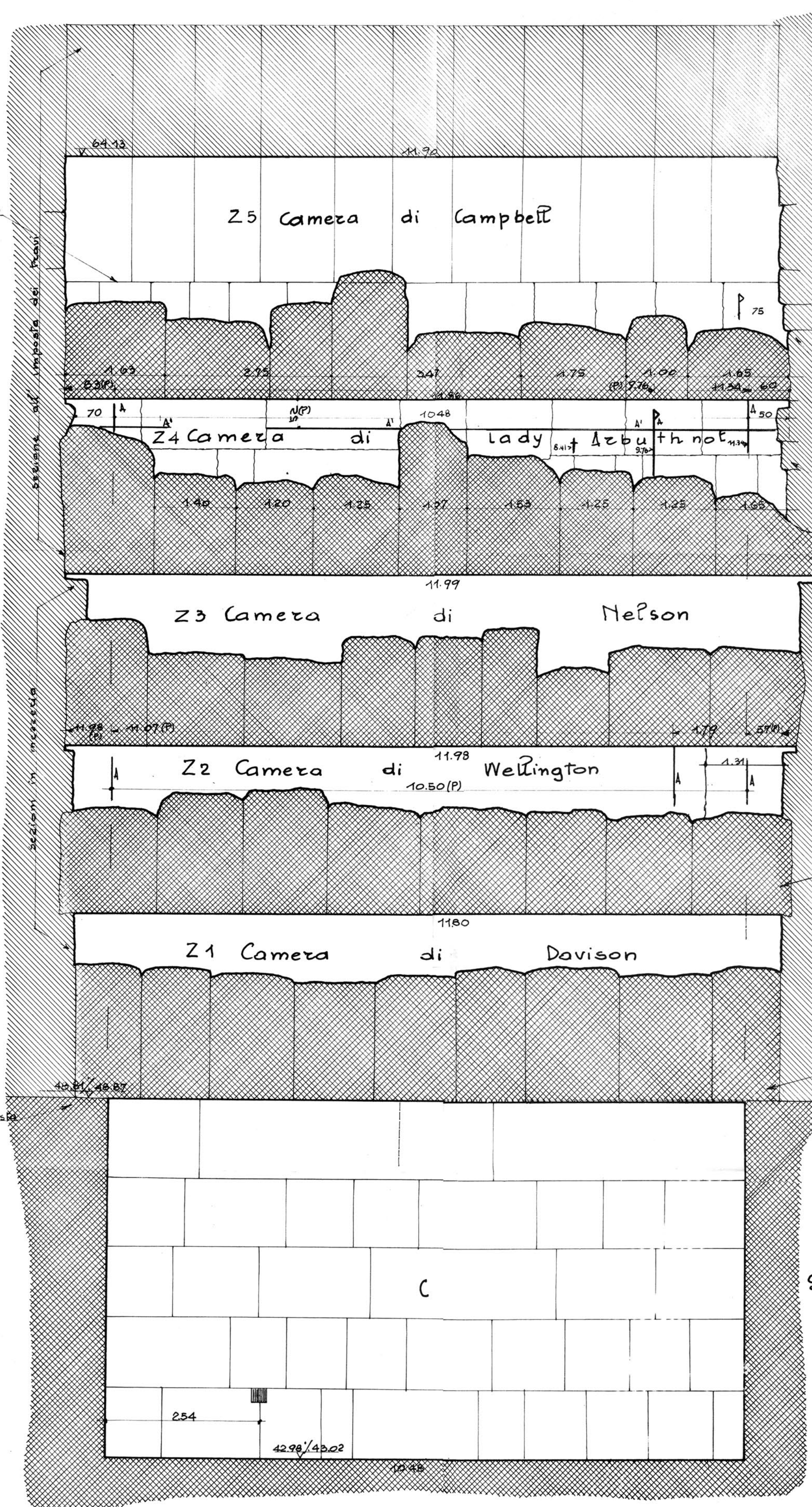
FIG. 1 SEZIONE E-W
