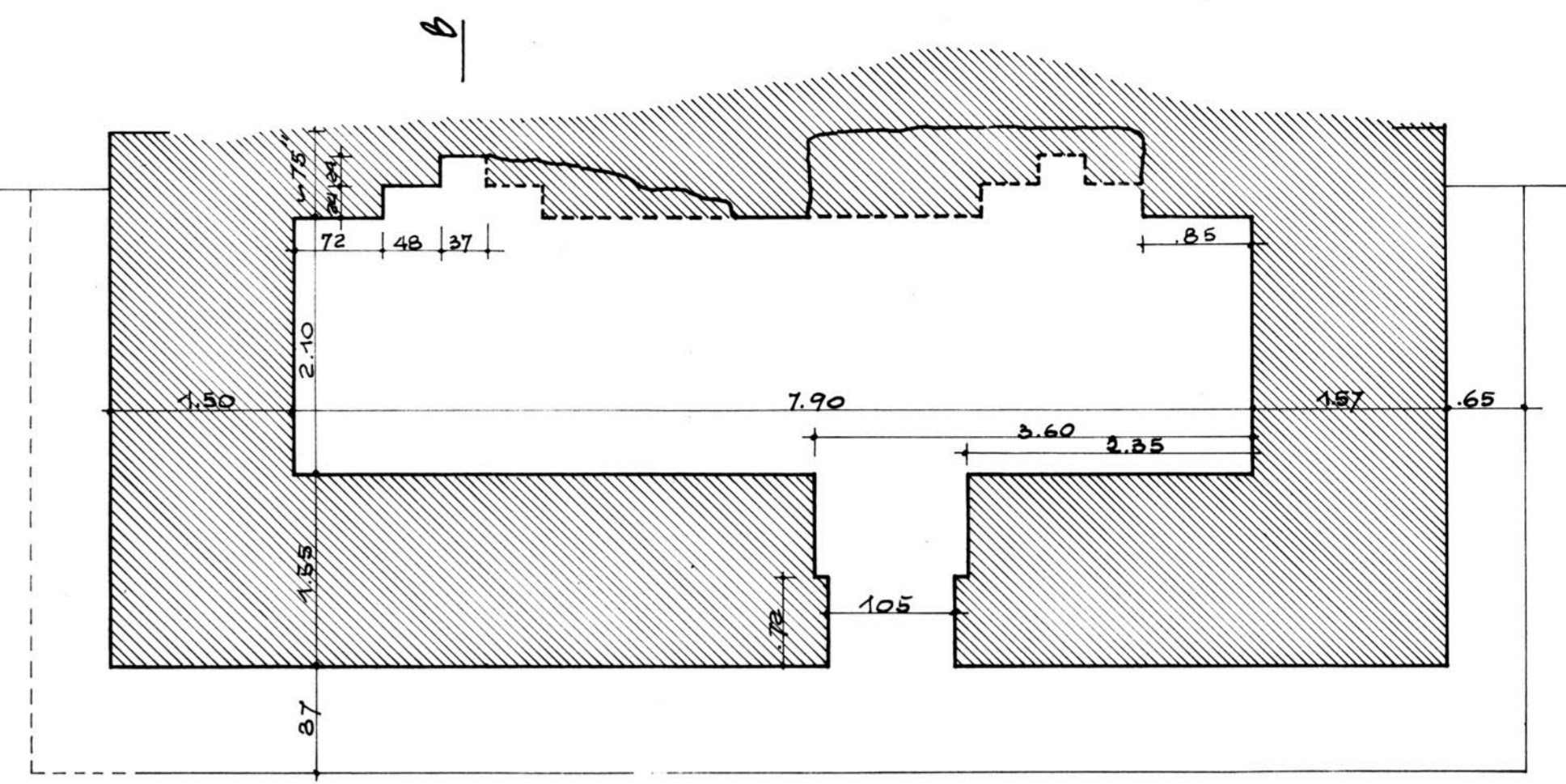
fig. 6 Pianta
