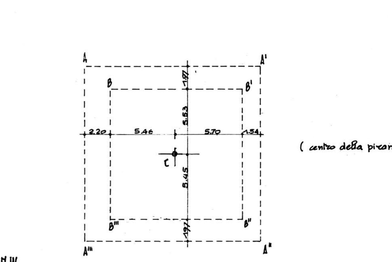
fig.12 PIATTAFORMA SUPERIORE (da Petrie)
