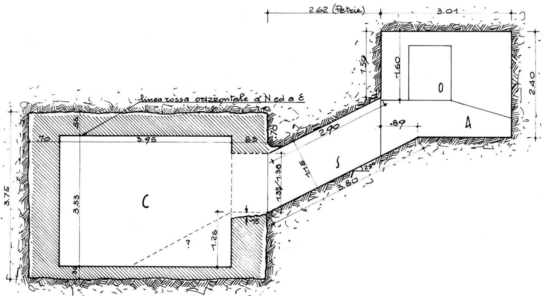
Fig. 4 Sezione E-W
