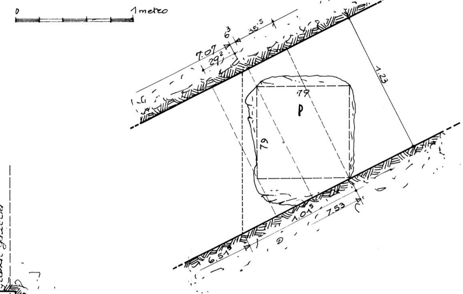
FIG. 2 PARTICOLARE DELLO SBICO INFERIORE DEL POZZO (Edgar)
