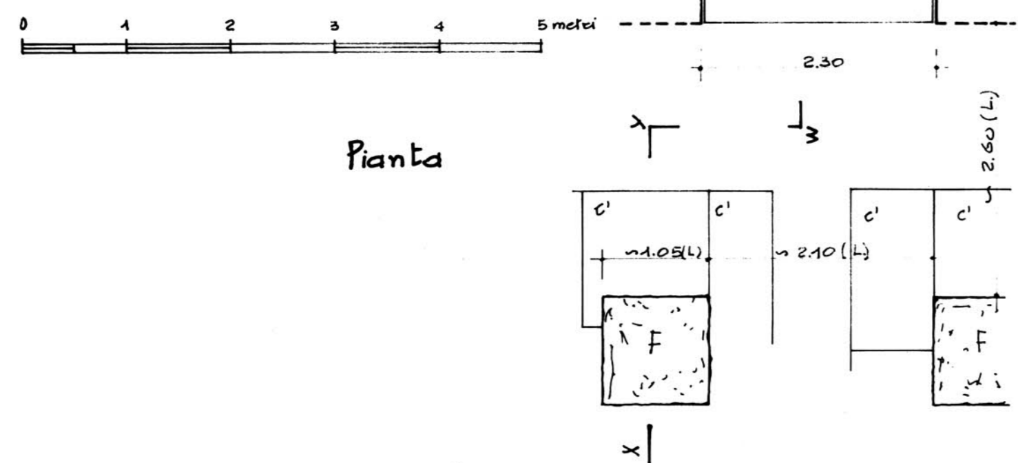
FIG. 4 PARTICOLARE DELLA PORTA Q
