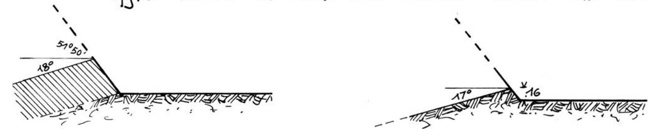
fig. 6 LETTO DI POSA DEL PRIMO CORSO AD EST
