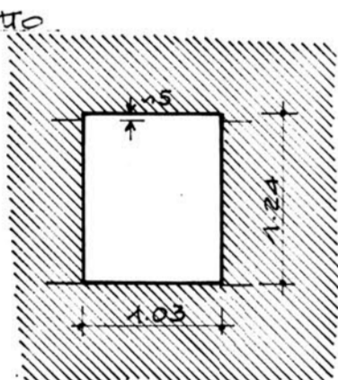
Fig. 2 Sezione della parte rivestita del corridoio discendente
