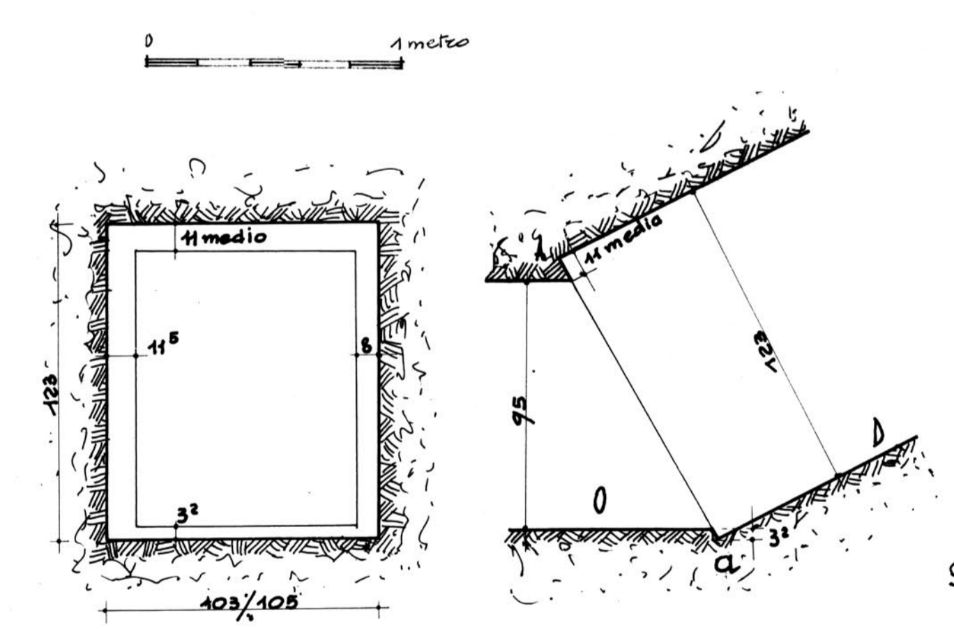
FIG. 3 PARTICOLARE DELLA SEZIONE A-a
