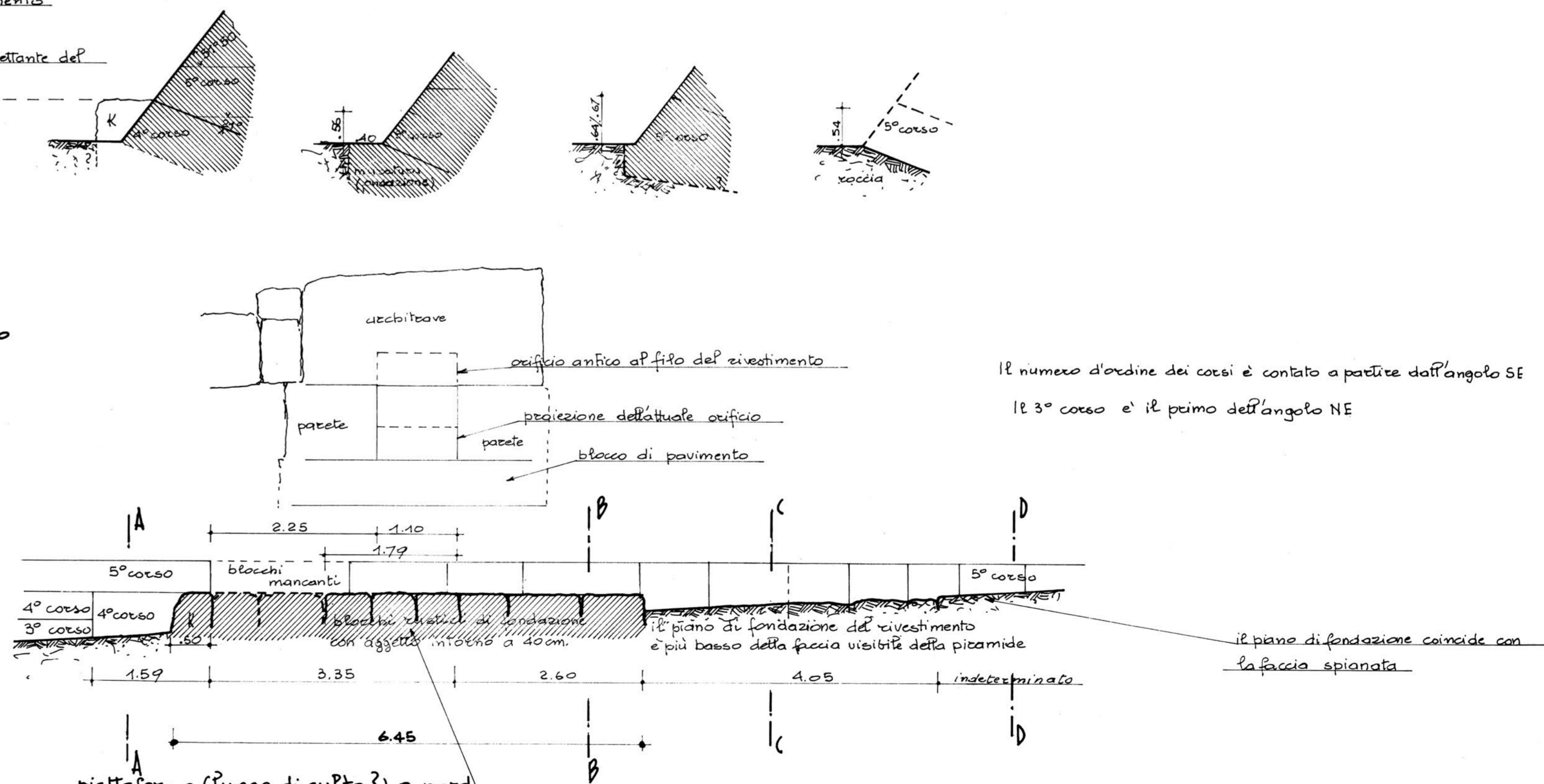
Fig. 6 SEZIONE LONGITUDINALE AL PIEDE DELLA FACCIA NORD
