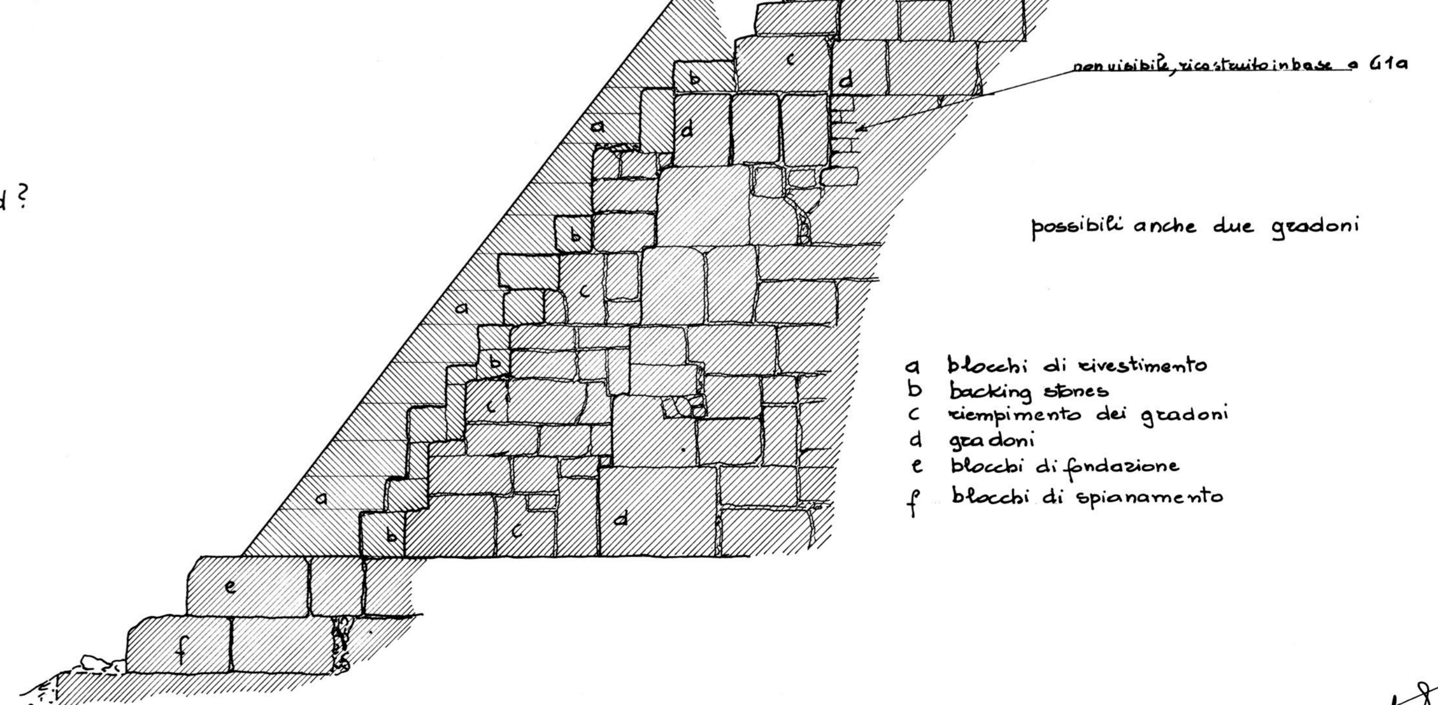
fig. 8 SCHEMA DELLA STRUTTURA (angolo SE)
