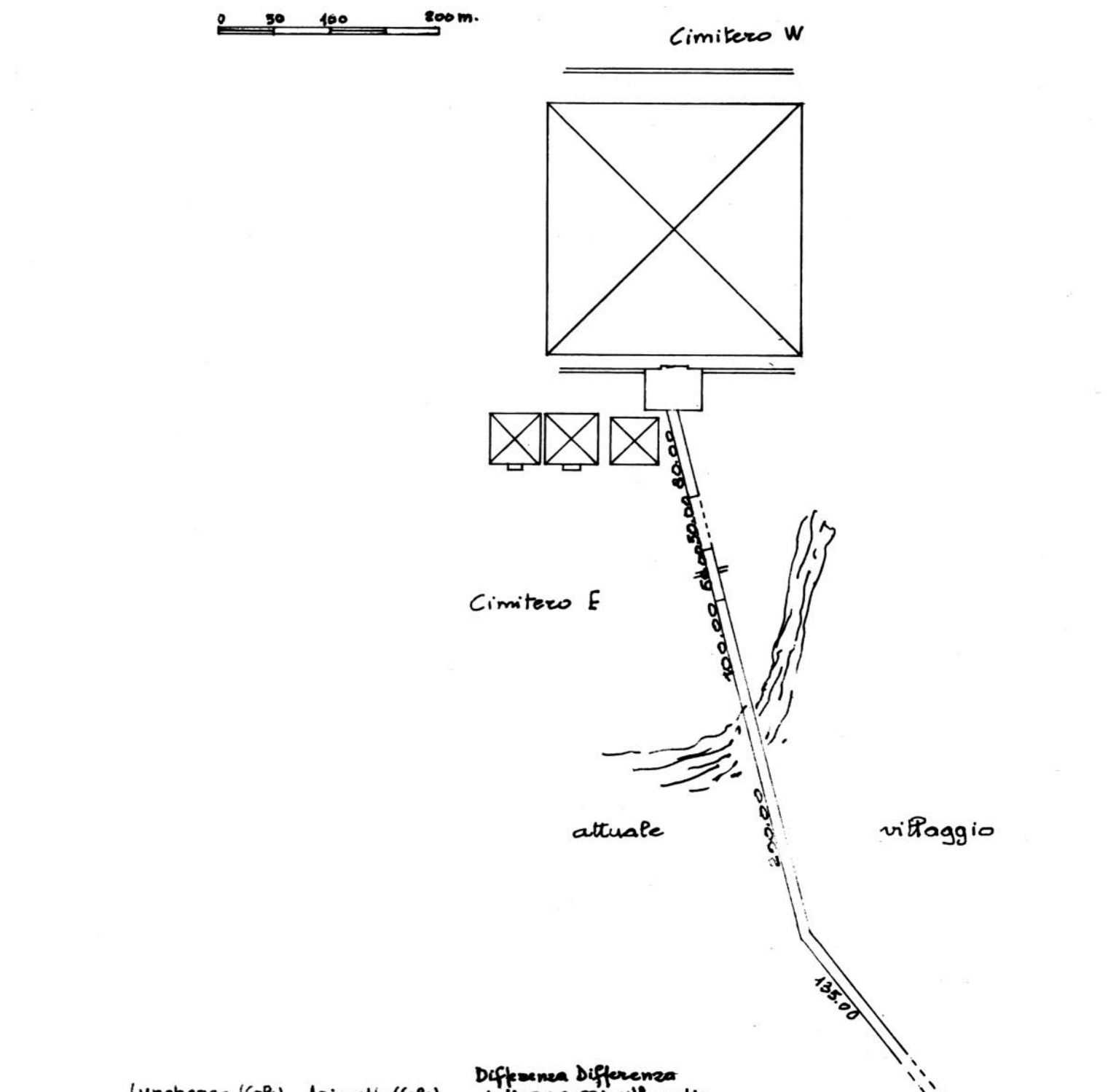
fig.2 DAMPA ALLA PIRAMIDE in base ai resti sull'altipiano ed ai rilievi di Flouing e di Lepsius
