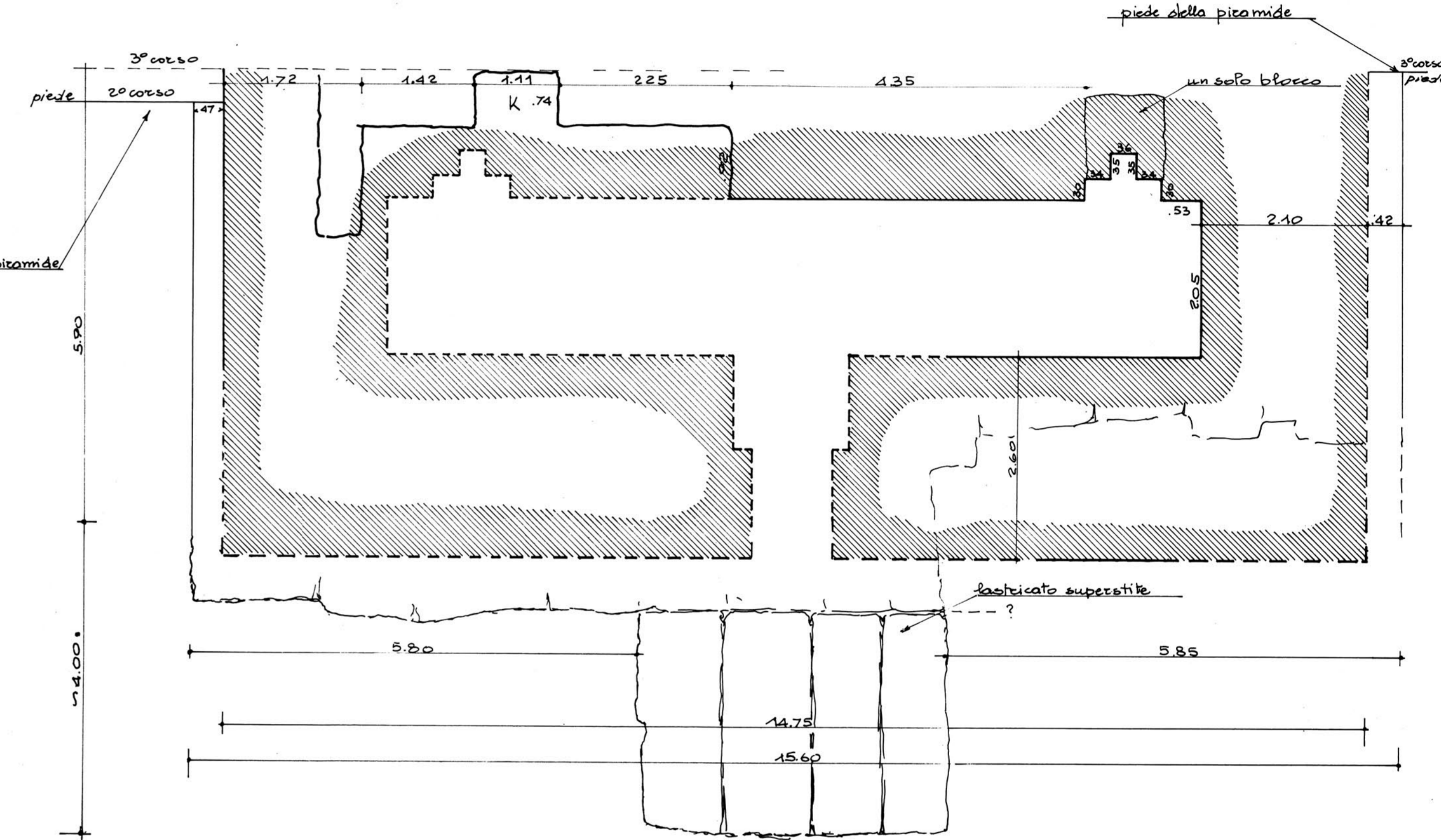
Fig. 5 SEZIONI TRASVERSALI ALLA FACCIA NORD
