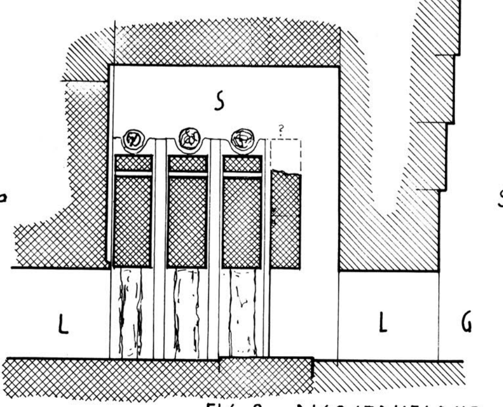
FIG. 8 RICOSTRUZIONE DEL SISTEMA DI CHIUSURA
