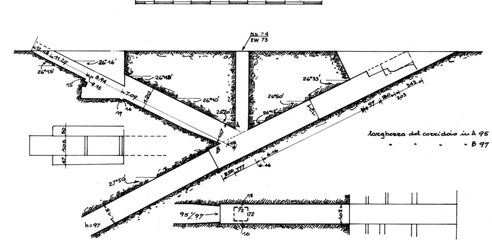
FIG. 6 TRIAL PASSAGE (Petrie)
