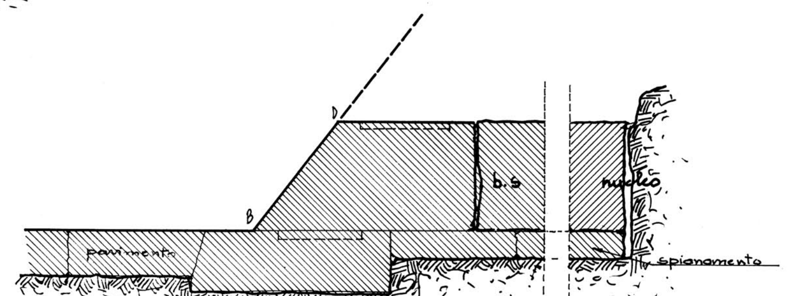
Fig. 16 Sezione AD secondo Borchardt (roccia)
