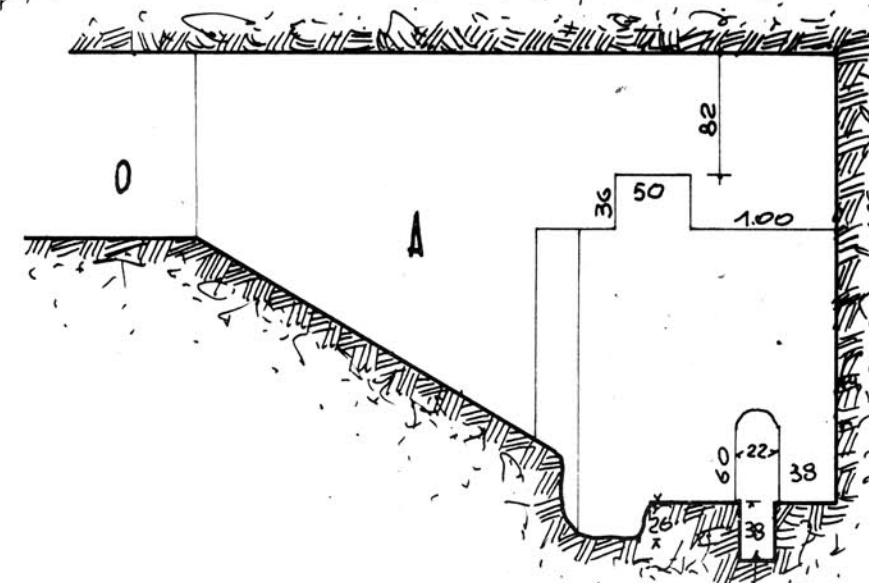
fig. 4 Elevazione ad Est della camera A
