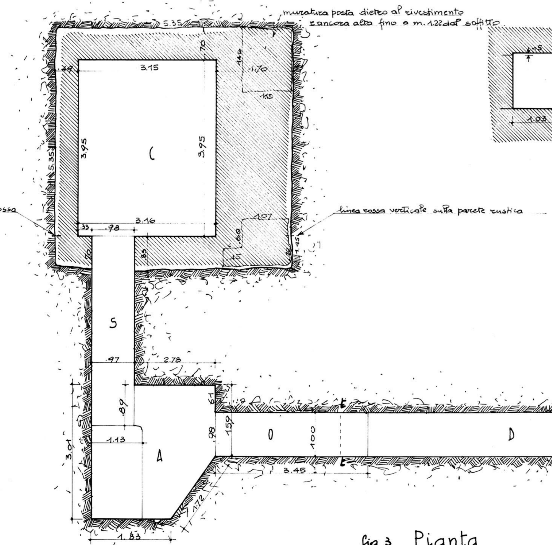
Fig. 3 Pianta
